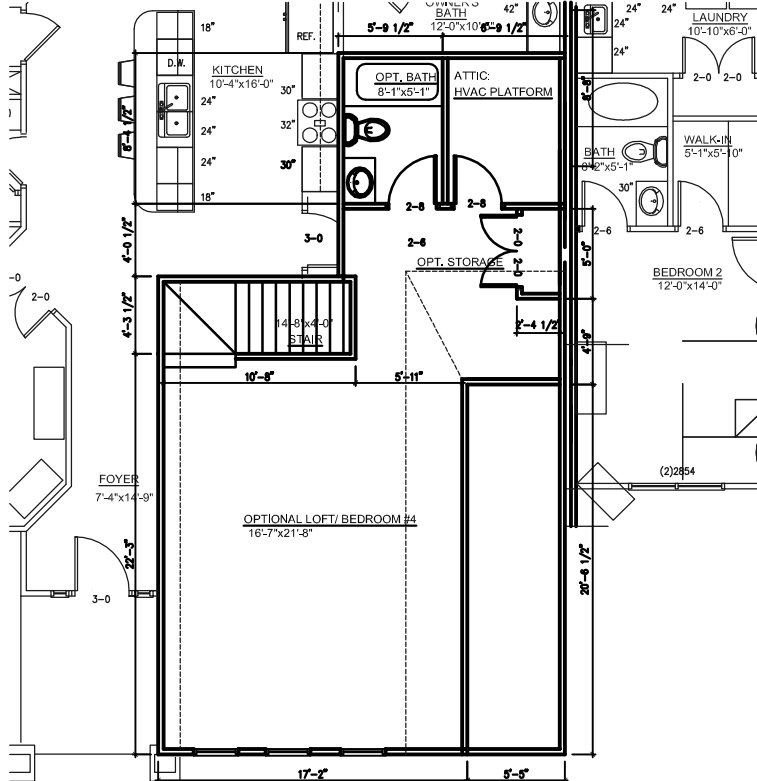
2 OPTIONAL LOFT
